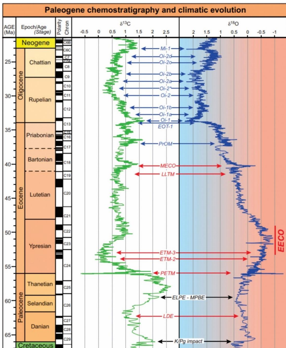
Fig. 3 Stabilirea și corelarea evenimentelor climatice în Scara stratigrafică, din Paleogen, pe baza variației izotopilor stabili de \delta^{13}C și \delta^{18}O (după Speijer et al., în Gradstein et al., edits., 2020).
